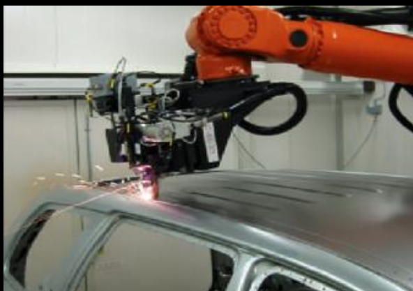
激光焊&激光切割
